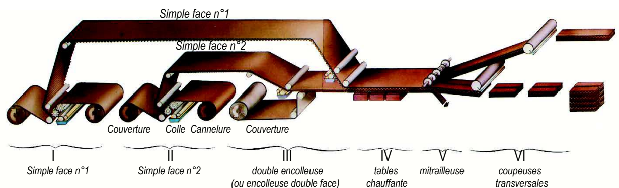
Fig. 3 – Fabrication du carton ondulé : vue générale schématique d'une onduleuse
