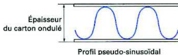
Fig. 2 – Profil de cannelure
