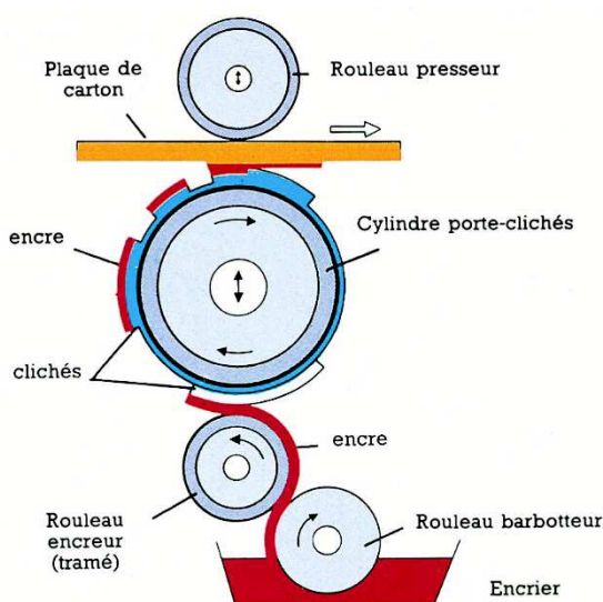
Fig. 7 – Flexographie
