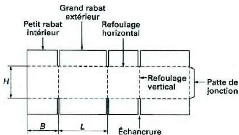
Fig. 10 – Caisses développées : différentes parties et cote de fabrication
