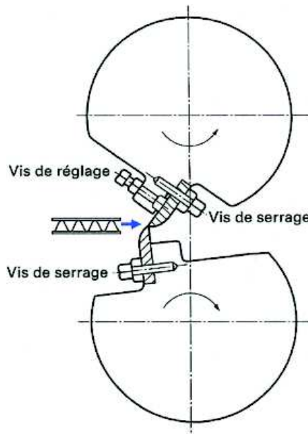
Fig. 6 – Coupeuse transversale
