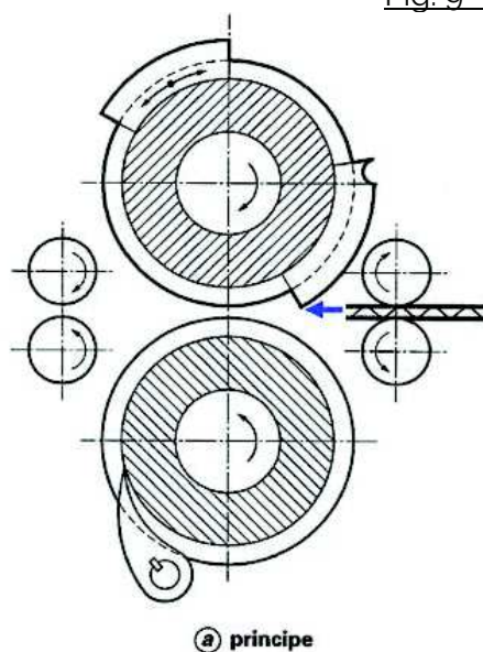
Fig. 9 – Slotter
