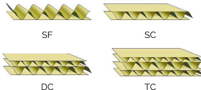
Fig. 1 – Principaux types de carton ondulé.
